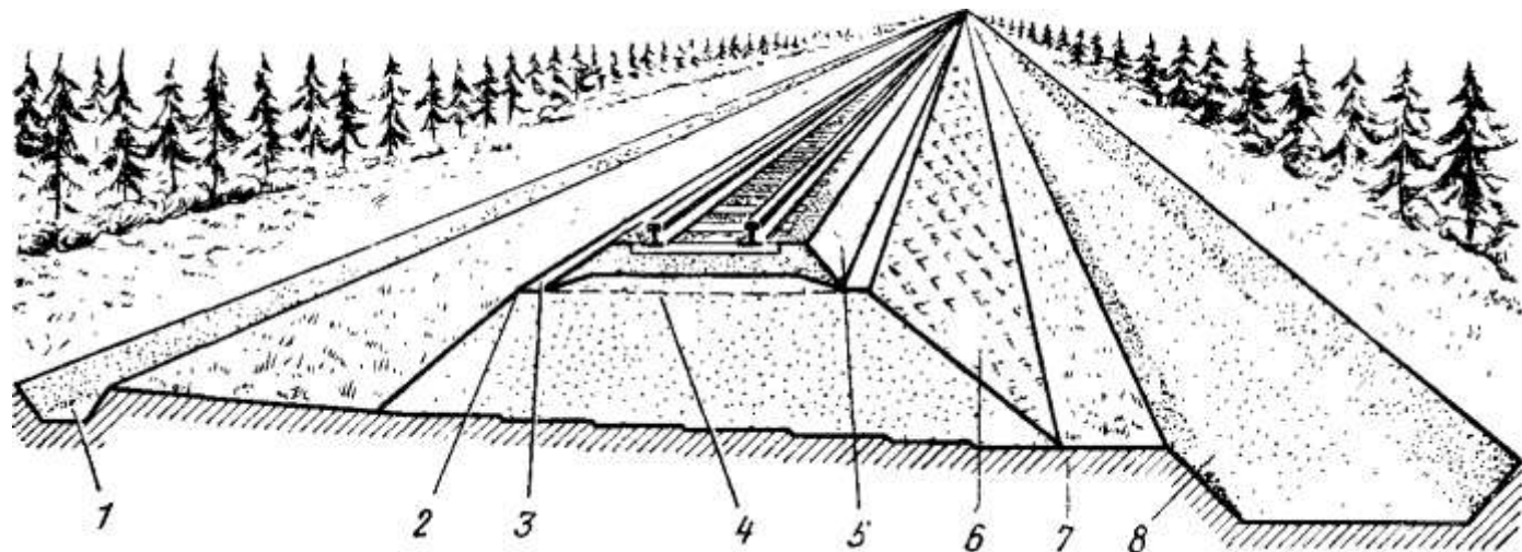
Поперечный разрез насыпи:
