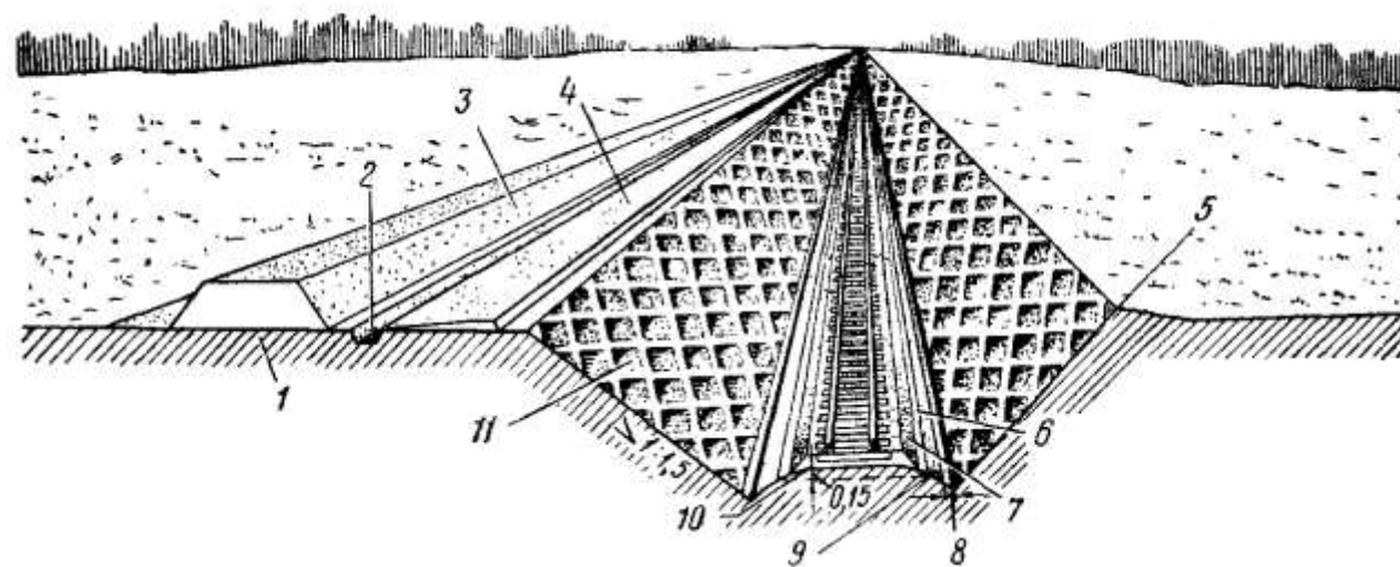
Поперечный разрез выемки:
